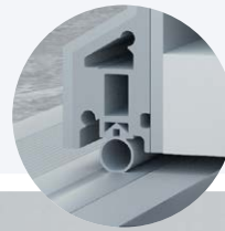
Abbildung: Verstellbare Silikon-Schleifdichtung
